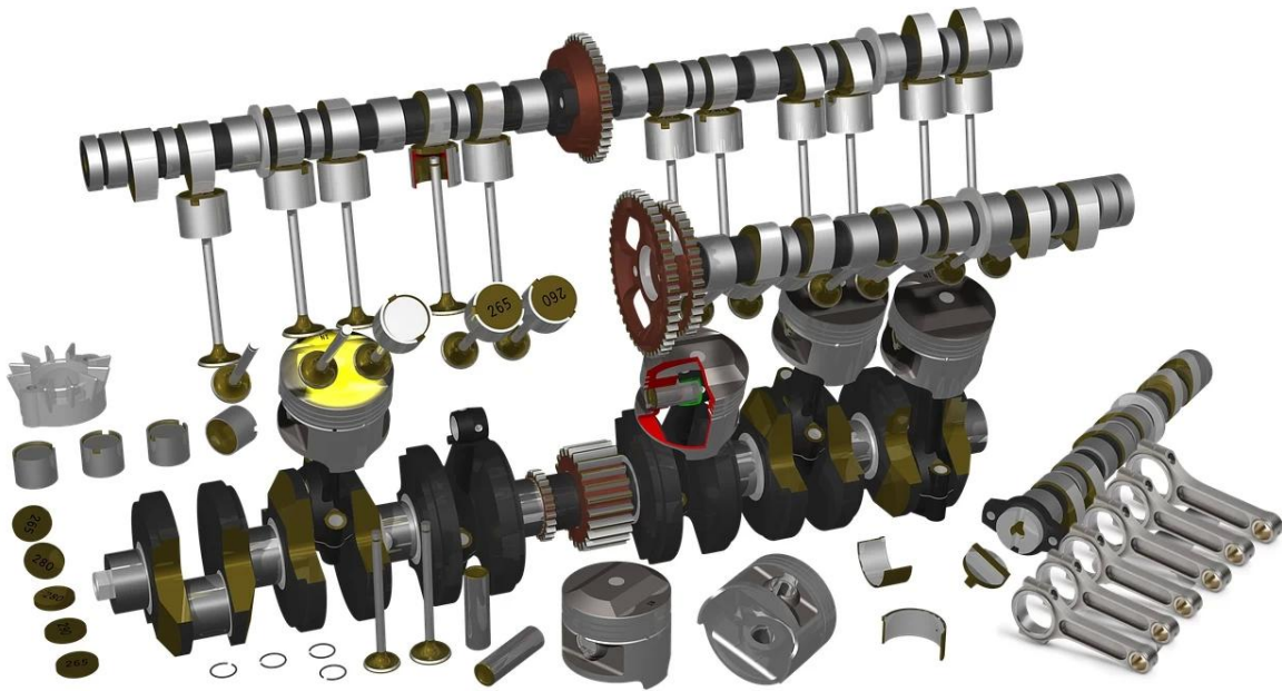
Vorgestelltes Produkt: HOLDEN L67 SUPERCHARGED 3.8L V6 - geschmiedete H-Träger-Pleuel aus 4340 Stahl
